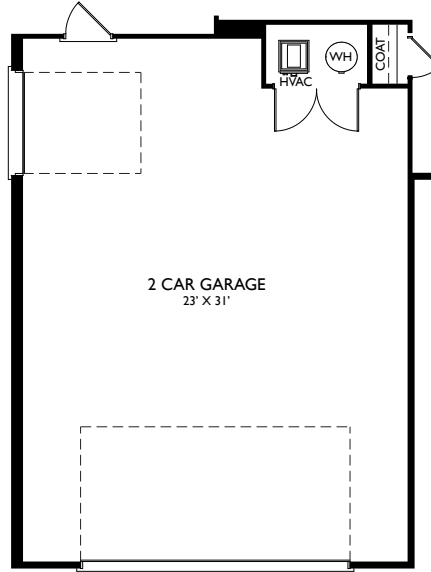
OPTIONAL GOLF CART GARAGE
